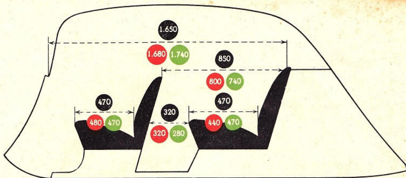
COUPE LONGITUDINALE
